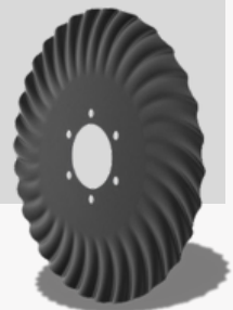
ON 33 AV 33 Ondulaciones Abertura de corte 7 mm.
