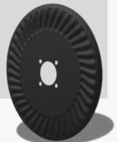
Tango Filo Liso. 40 Ondulaciones. Abertura de corte 9 mm.
